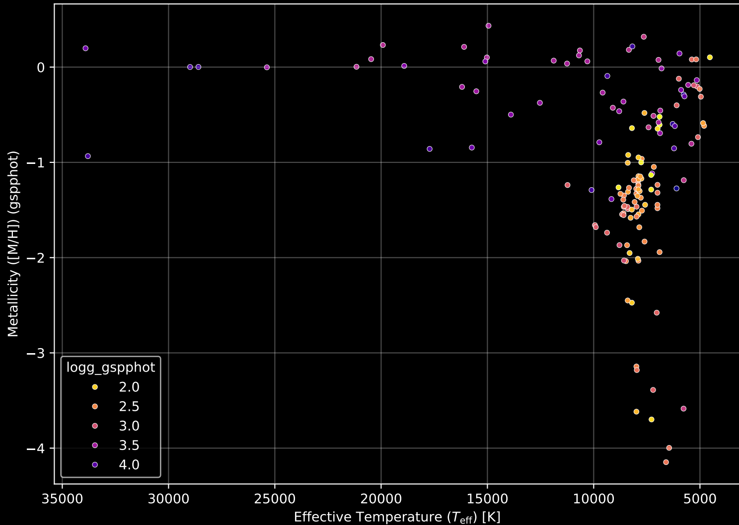
APOGEE DR17 Field: [291-00-C] Stellar Population Parameters (n= 149)
